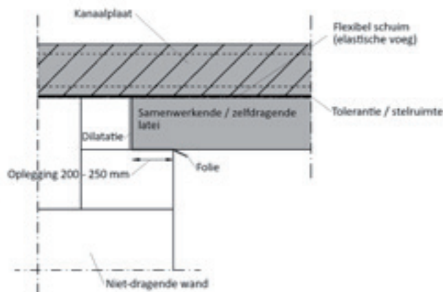
Latei niet-dragende wand
