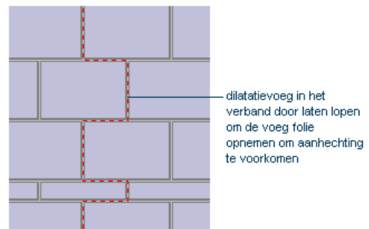
Dilatatievoeg in een niet-dragende wand op een gefundeerde ondergrond
