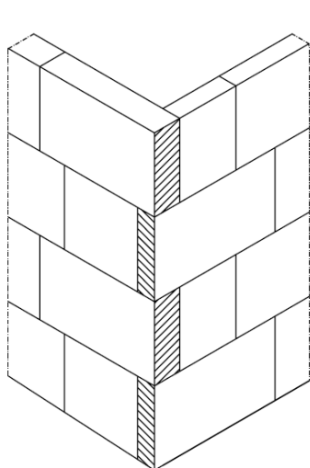
Vertande hoekaansluiting
